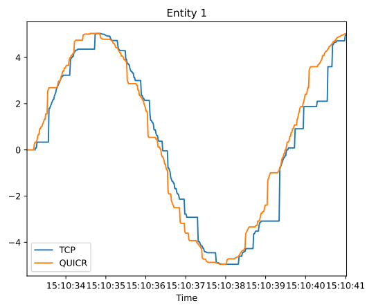
Obrázek 20: Porovnání TCP a QUICr v peer-to-peer
