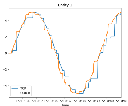
Obrázek 21: Porovnání TCP a QUICr v peer-to-peer
